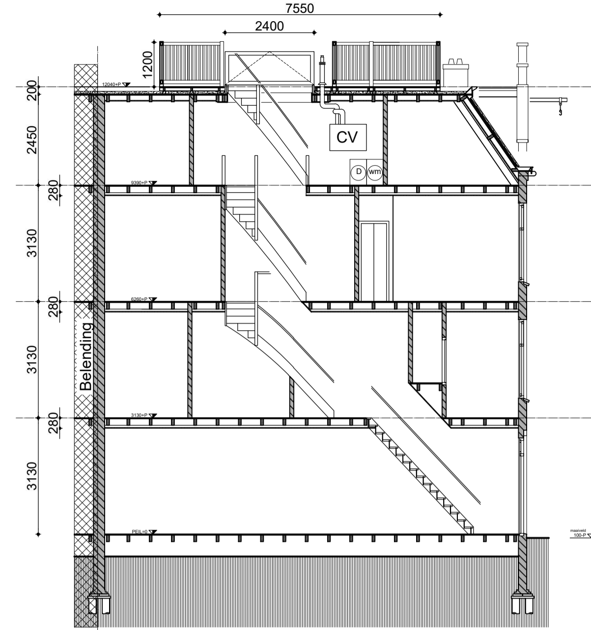
Langsdoorsnede A-A
