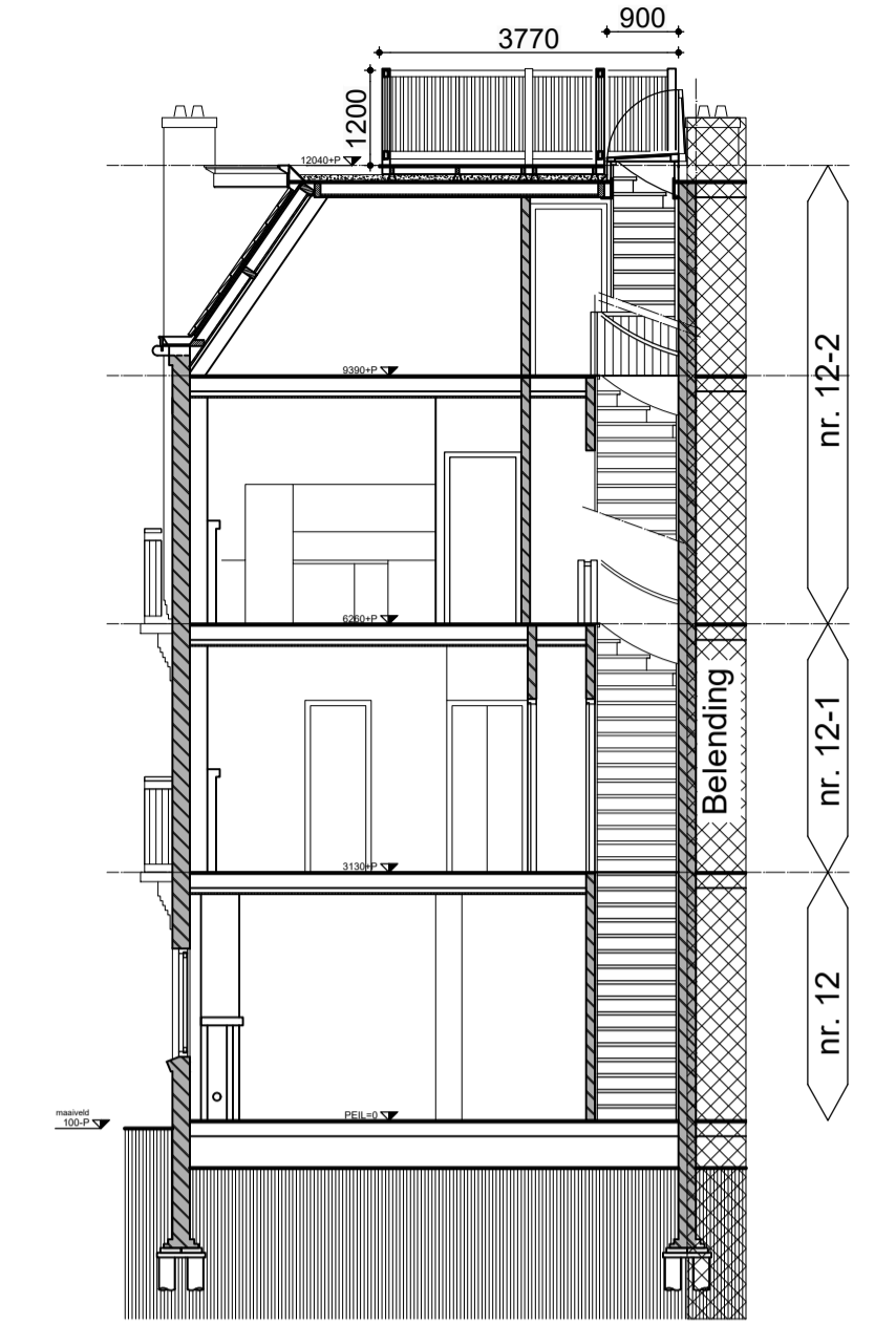
Dwarsdoorsnede B-B
